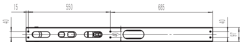
下导轨安装面
